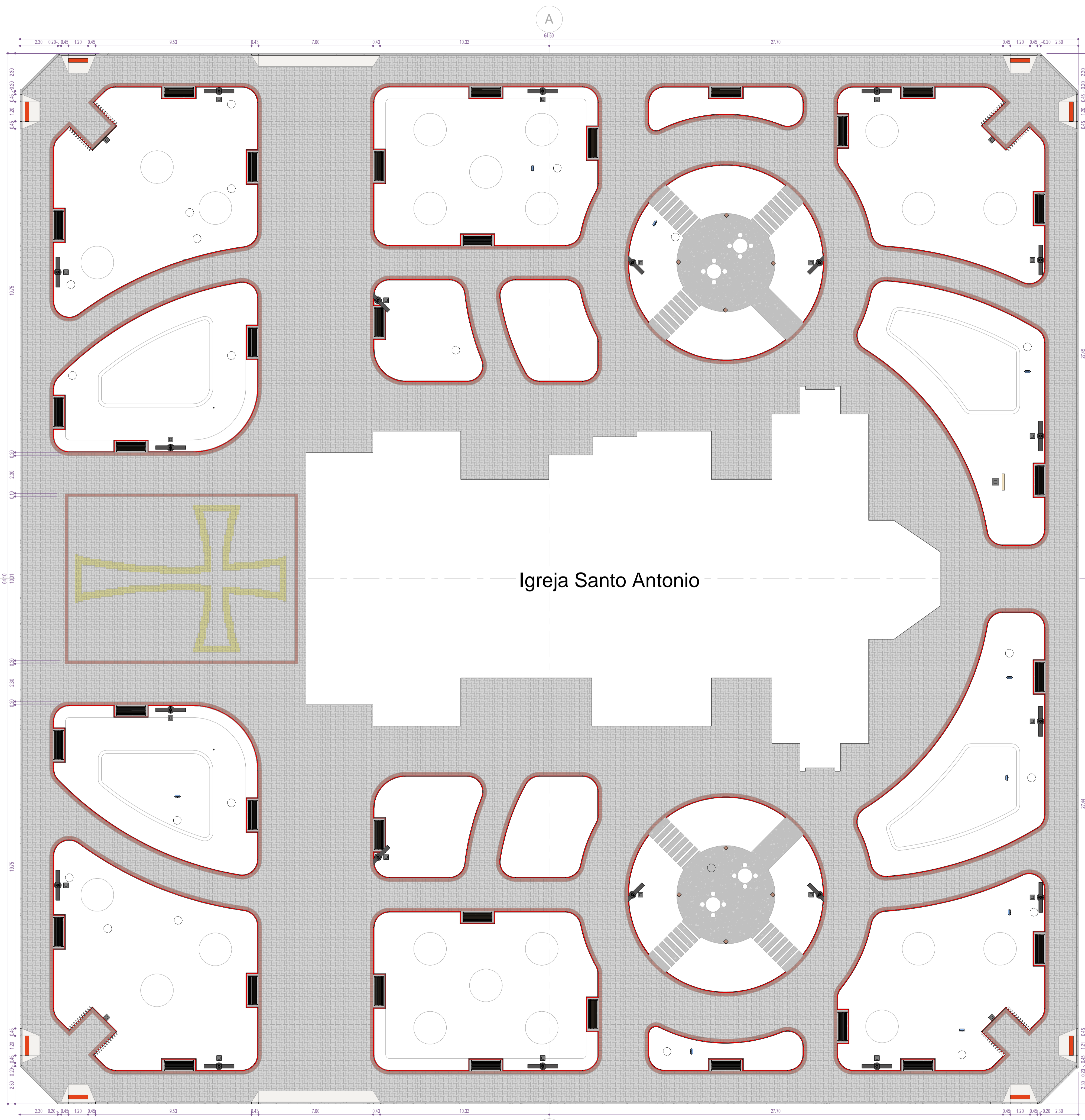
1 Planta de Pisos 1 : 125
