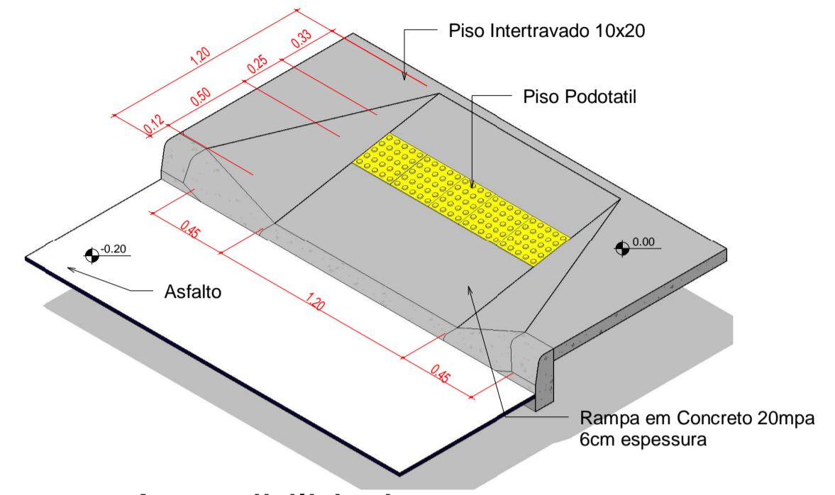
4 Vista 3D - Rampa Acessibilidade
